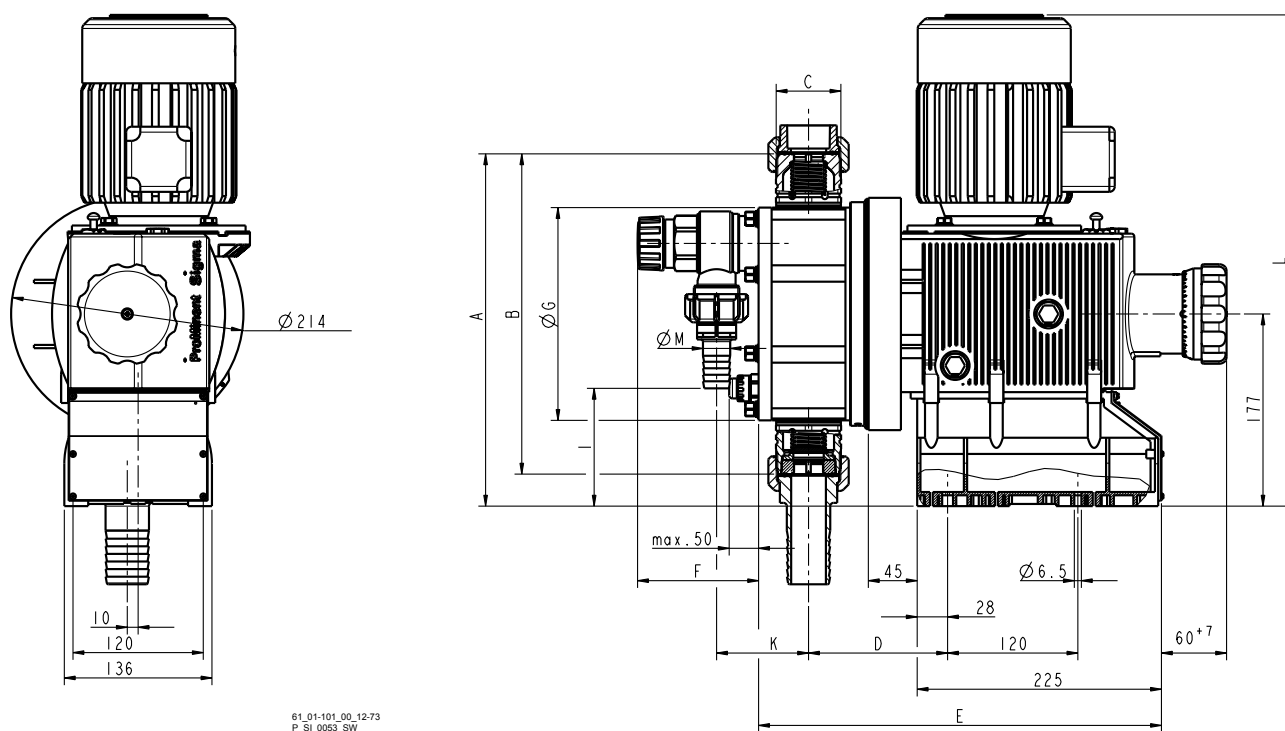
Fig. 27 : Dessin coté Sigma/ 3, S3Ba - Cotes en mm - Présentation non contractuelle.
