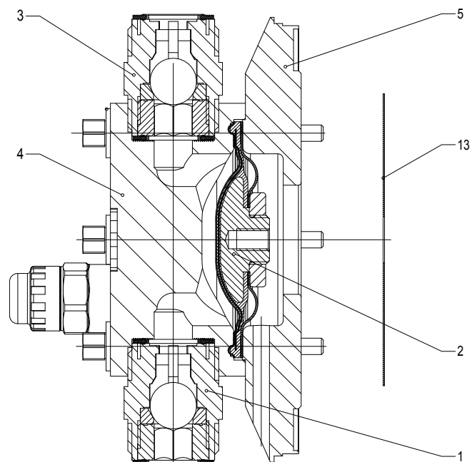
Fig. 7 : Vue en coupe de l'unité de refoulement
