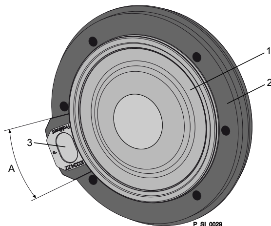
Fig. 23 : Zone de tolérance de la languette sur l'entretoise de la tête
