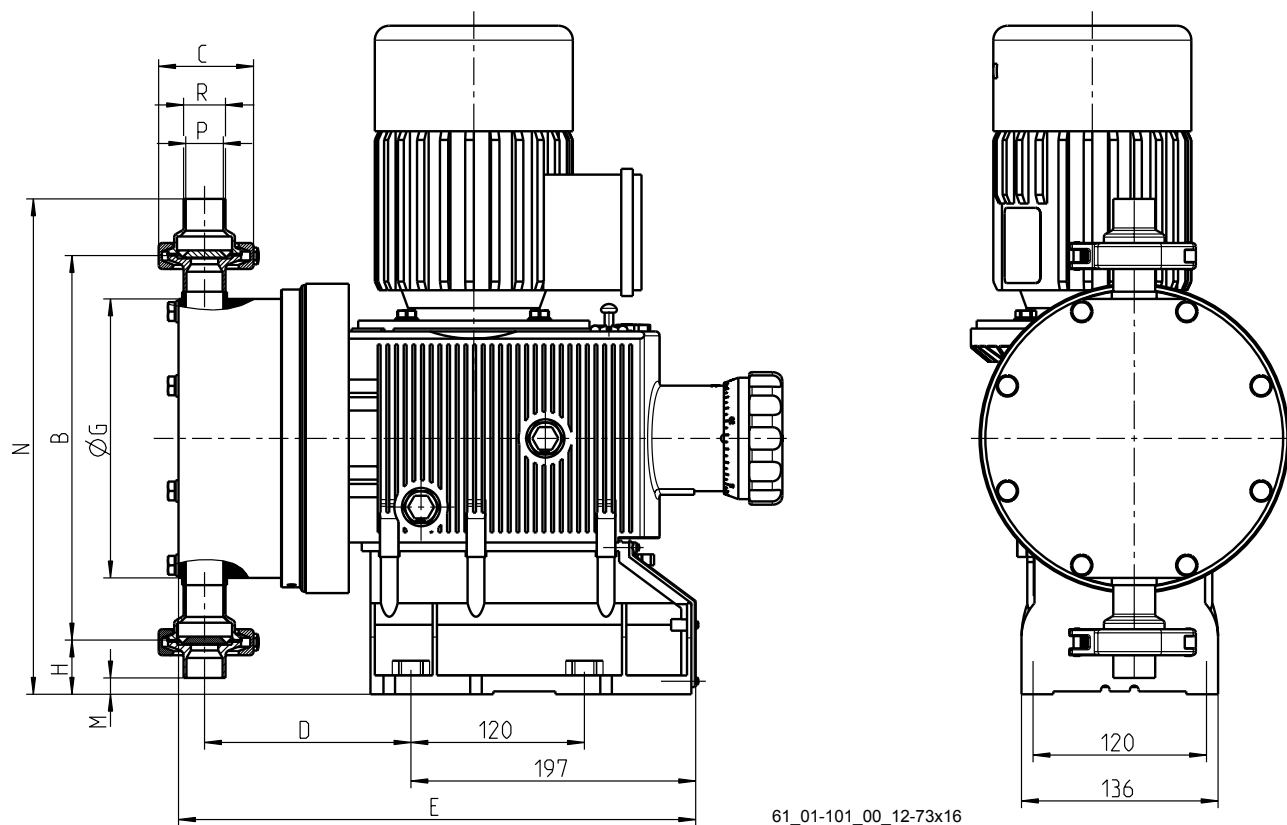
Fig. 29 : Dessin coté Sigma/ 3, S3Ba, avec module de dosage « physiologiquement neutre » - Cotes en mm - Présentation non contractuelle.
