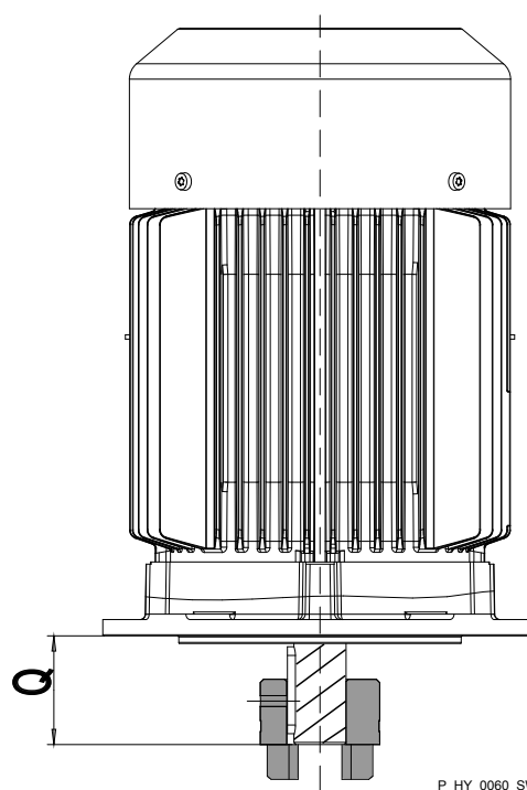
Fig. 10 : Hauteur correcte de la griffe de l'accouplement sur l'arbre moteur
