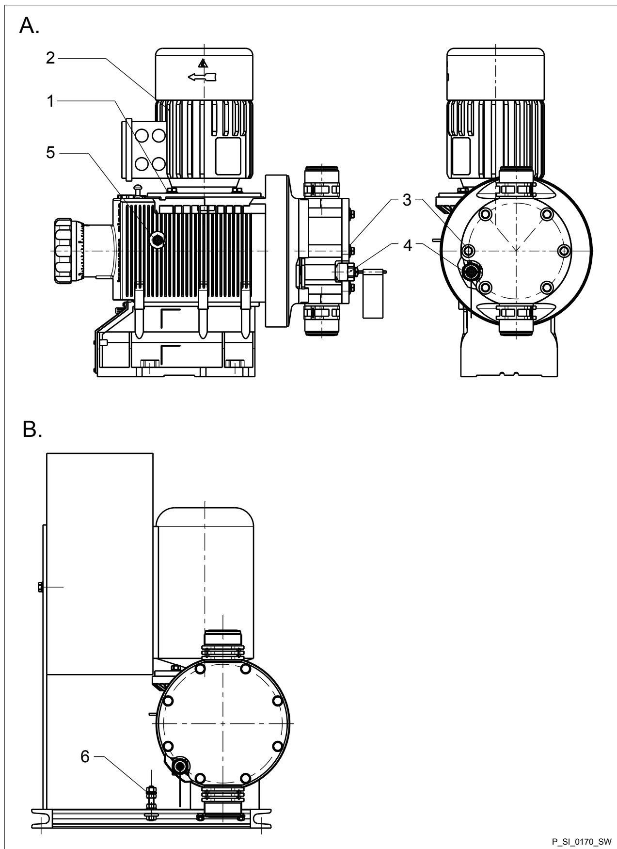
Fig. 31 : Plans de compensation de potentiel Sigma S3Ba; A. Pompe sans cadre, B. Pompe avec cadre
