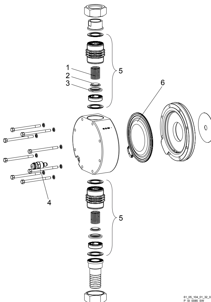
Fig. 37 : Module de dosage Sigma/ 3 1000 SST
