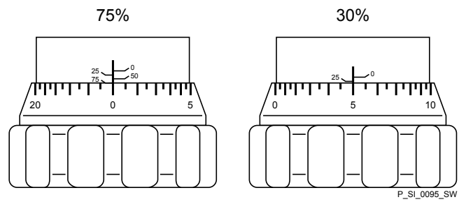
Fig. 5 : Régler la longueur de course
