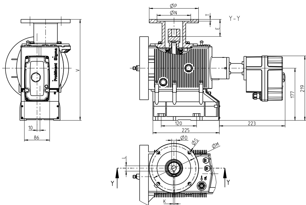
Fig. 28 : Dessin coté Sigma/ 3, S3Ba avec bride moteur - Cotes en mm - Présentation non contractuelle.
