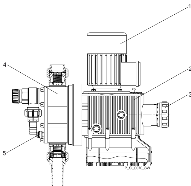
Fig. 3 : Présentation de l'appareil et éléments de commande S3Ba
