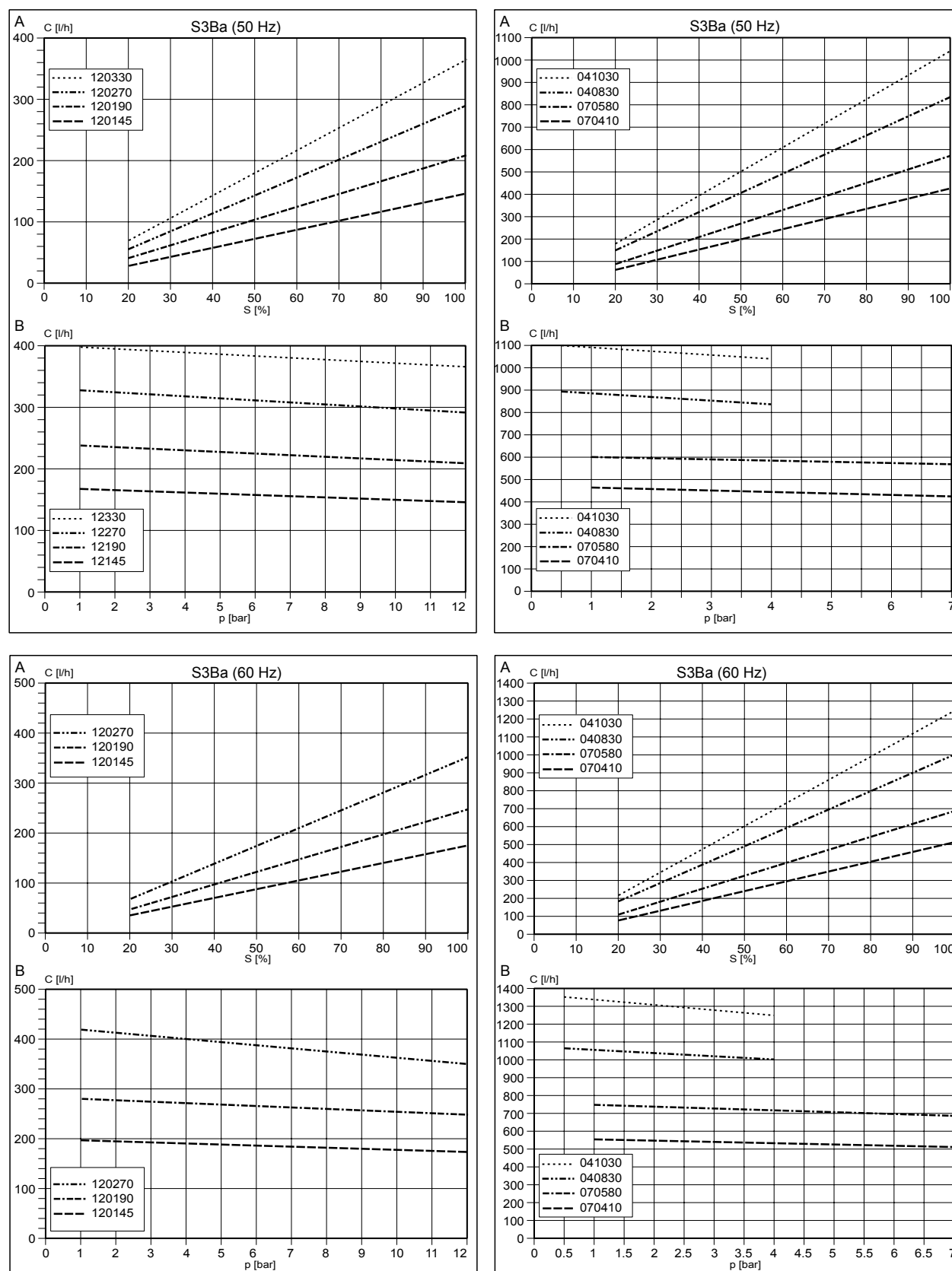
Fig. 26 : A) Débit de dosage C à la contre-pression minimale en fonction de la longueur de course, voir B) Débit de dosage C à la contre-pression p .
