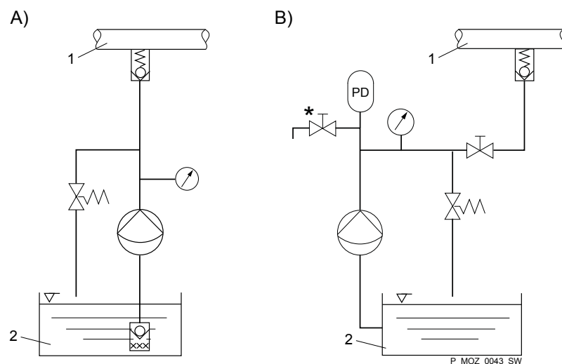
Fig. 18 : A) Installation standard, B) Avec amortisseur de pulsations
