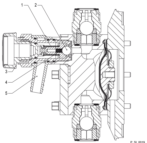
Fig. 8 : Soupape de décharge intégrée
