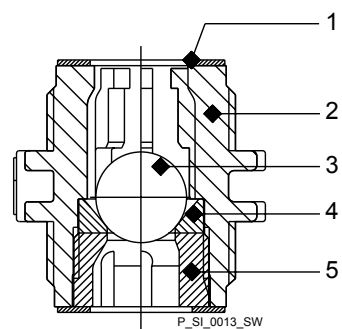
Fig. 22 : Clapet à bille unique, vue en coupe
