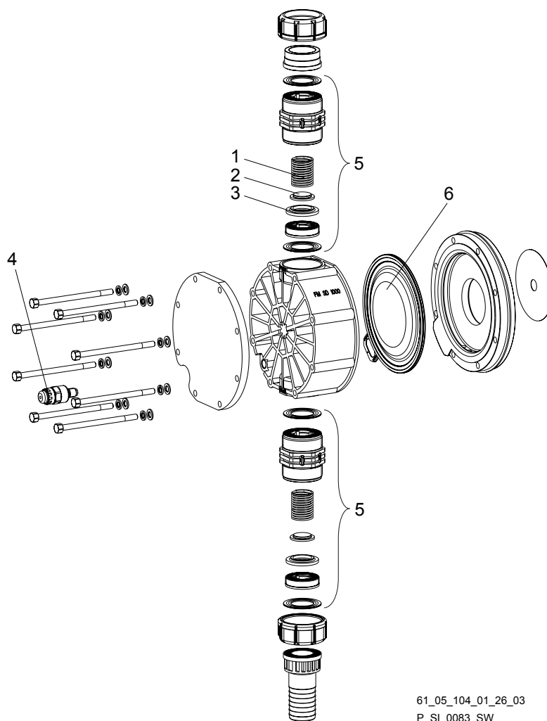
Fig. 33 : Module de dosage Sigma/ 3 1000 PVT
