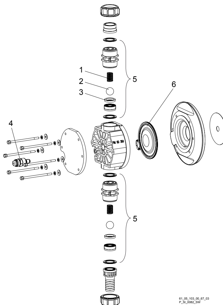
Fig. 32 : Module de dosage Sigma/ 3 330 PVT
