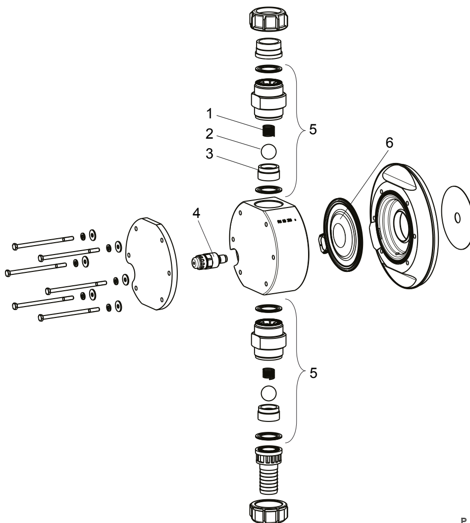
Fig. 35 : Module de dosage Sigma/ 3 330 TTT
