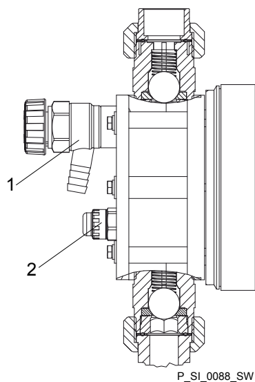
Fig. 4 : Éléments de commande Sigma
