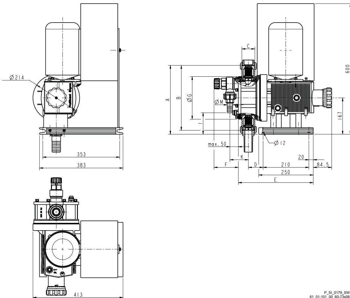
Fig. 30 : Dessin coté Sigma/ 3, S3Ba, avec moteur ATEX-FU - Cotes en mm - Présentation non contractuelle.
