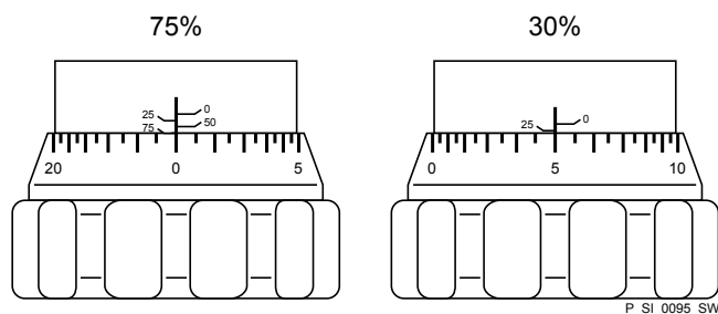
Fig. 20 : Réglage de la longueur de course
