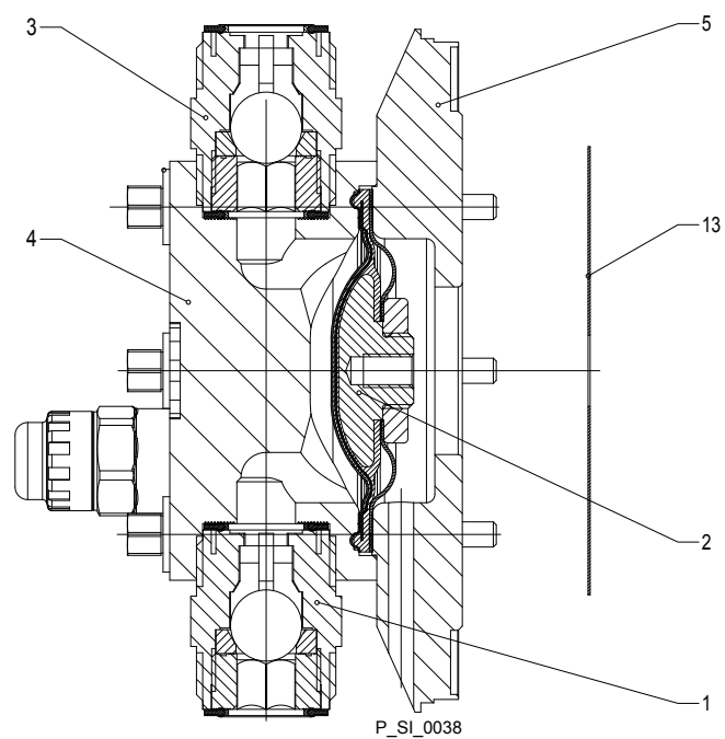
Fig. 25 : Vue en coupe du module de dosage
