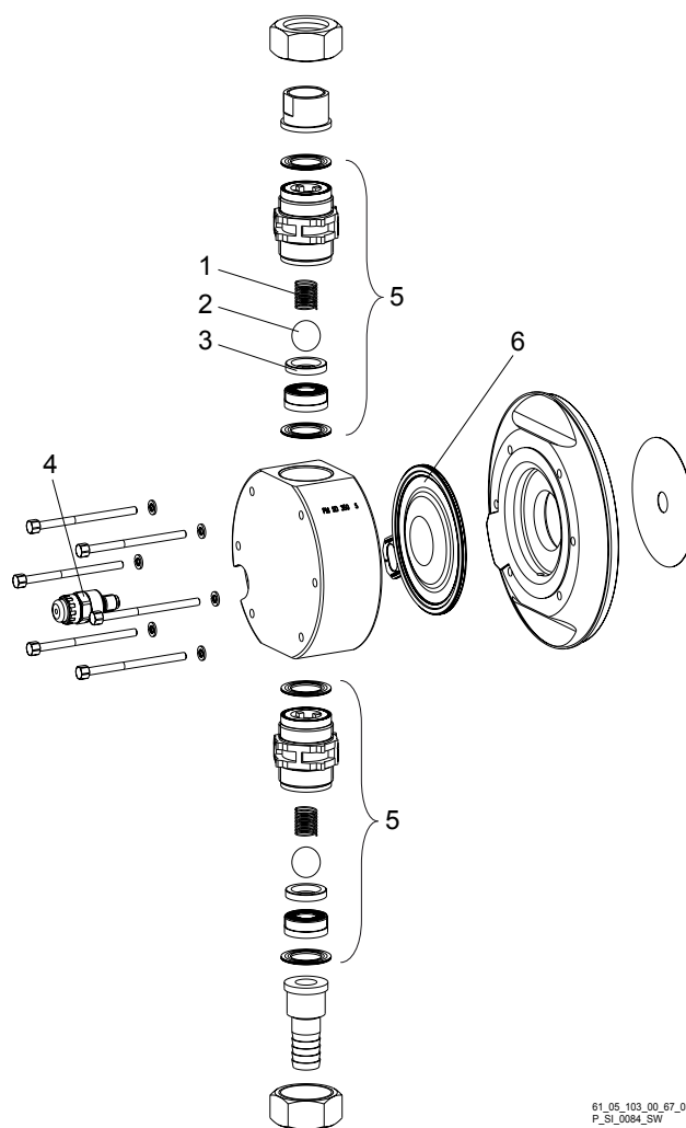
Fig. 36 : Module de dosage Sigma/ 3 330 SST
