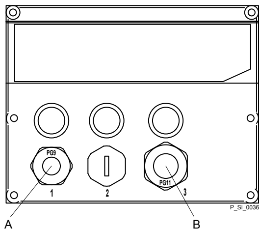
Fig. 6 : Couvercle frontal sur l'exécution avec relais tact
