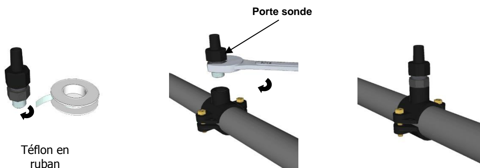
Porte sonde
