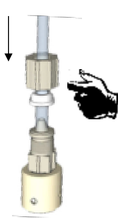
Etape 12 Dévisser le bouchon et passer le tube clair.
