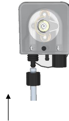
Etape 17 Visser le tube PVC (Transparent) sur la pompe doseuse.
