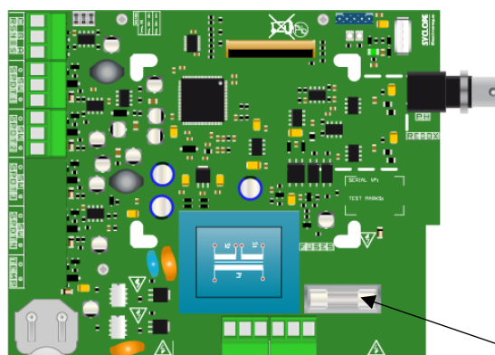
Fusible verre 5x20 250mA Temporisé
